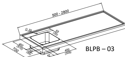
Panneau avec égouttoir, bac et trou pour pompe à bière
