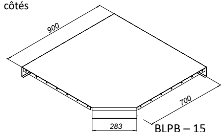
Panneau d'angle 45° – extérieur – lié de deux côtés
