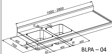
Panneau avec deux bacs et égouttoir
