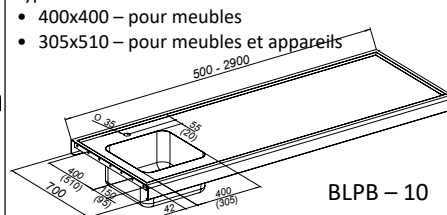
Panneau pour meuble à bouteilles – lié de deux côtés
