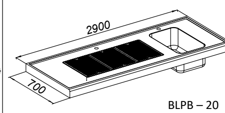
Panneau avec bac 307x510 et large égouttoir lié d'un côté type P (L)
