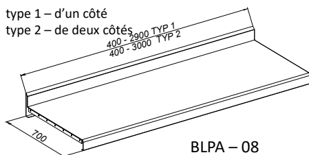
Panneau avec décaissé partiel et bac
