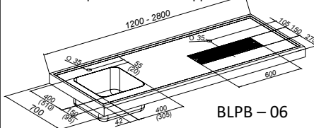
Panneau avec décaissé lié
