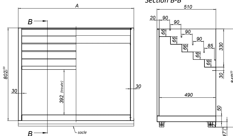
Soubassement à bouteilles BLN-0008
