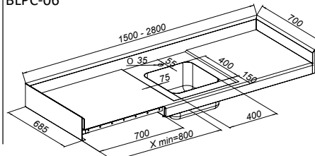
Panneau avec décaissé partiel et bac 400x400, lié d'un côté – type L (P)
