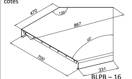
Panneau pour meuble à bouteilles – lié d'un côté
