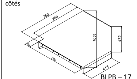
Panneau avec bac 307x510 et large égouttoir lié d'un côté type P (L)
