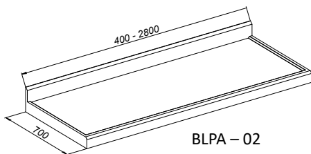
Panneau avec égouttoir
