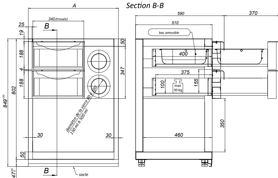
Soubassement étuve avec distributeur de verres et tiroir BLN-0010
