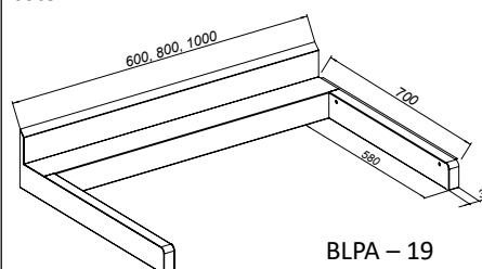
Panneau pour armoire à bouteilles – lié d'un côté
