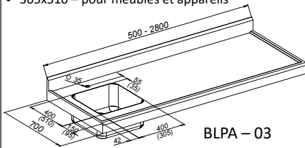
Panneau avec égouttoir, bac et trou pour pompe à bière
