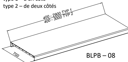
Panneau avec décaissé partiel et bac
