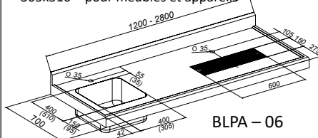
Panneau avec décaissé lié
