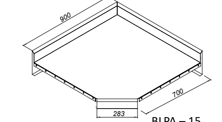
Panneau d'angle 45° – extérieur – lié de deux côtés
