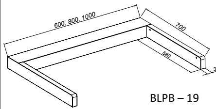
Panneau pour meuble à bouteilles – lié d'un côté
