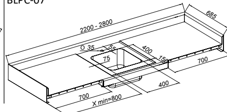
Panneau avec décaissé partiel et bac 400x400 – lié de deux côtés
