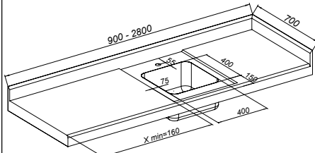
Panneau avec décaissé partiel et bac 400x400 – lié d'un côté
