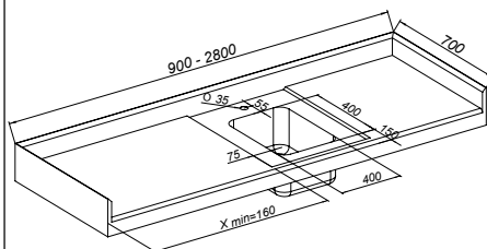
Panneau avec décaissé partiel et bac 400x400, lié d'un côté – type L (P)
