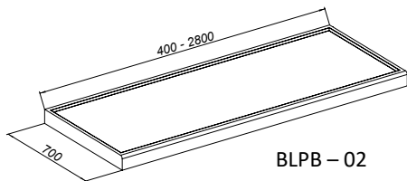
Panneau avec égouttoir et trou pour pompe à bière
