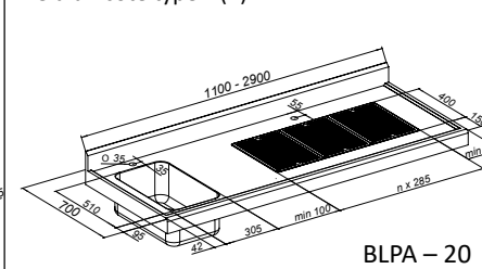
Panneau avec bac 307x510 et large égouttoir lié d'un côté type L (P)
