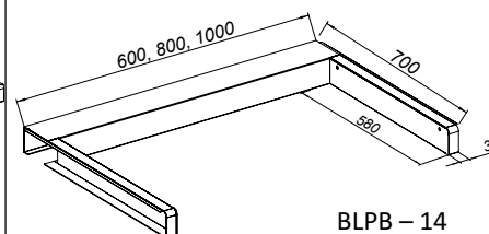
Panneau d'angle 90° – extérieur – lié de deux côtés
